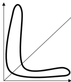
سیستم پایدار
