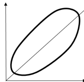
سیستم ناپایدار
