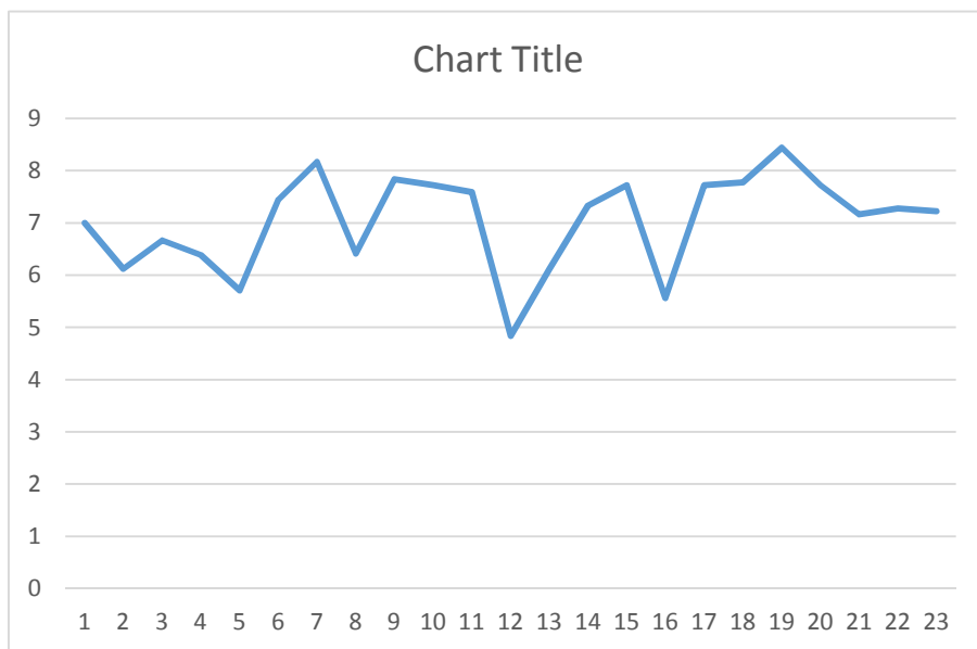
شکل ۴- مجموع ۲۳ شاخص
